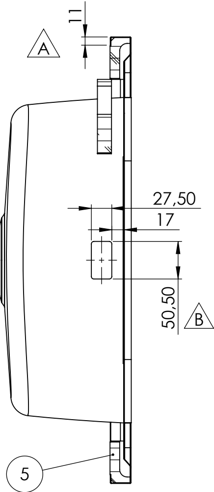
SECTION A-A
