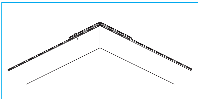
Tätning vidnock
